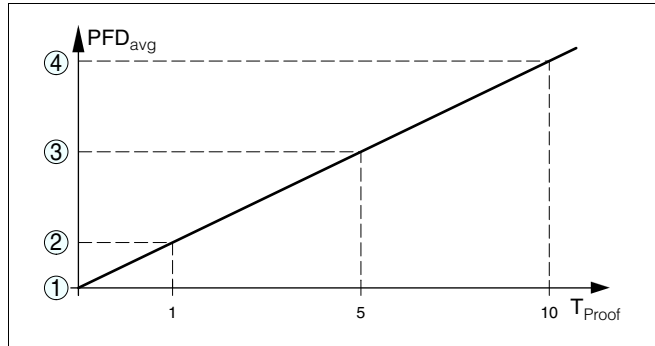
Fig. 1: Déroulement en fonction du temps de PFD_{avg} (valeurs numériques voir tableaux représentés ci-dessus)
