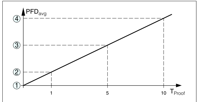
Abb. 1: Zeitabhängiger Verlauf von PFD_{\text{avg}} (Zahlenwerte siehe oben dargestellte Tabellen)
